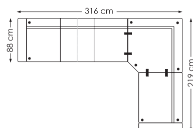
VILLA Oppsett L Arm-3,5 s-90 hj.-1,5 Big s-Arm Vendbar
